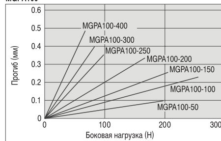
MGPA100
