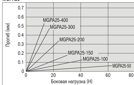
MGPA25
