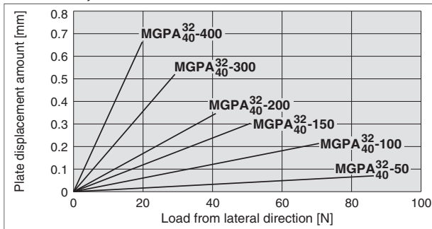
MGPA32, 40
