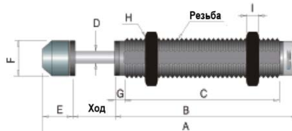
С упорным колпачком
