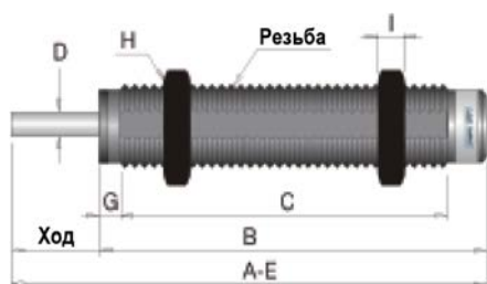
Без упорного колпачка
