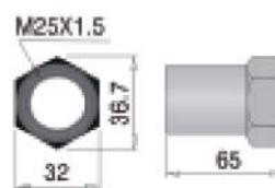
RSC25-2-XLC01
