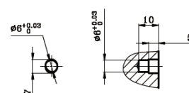
Вид на отверстия G
