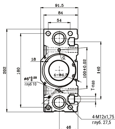
Вид на Т-образный паз
