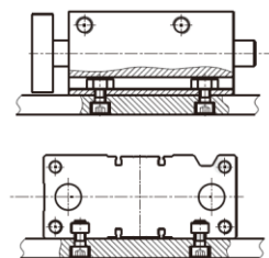
Фиксация за паз снизу
