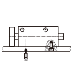
С помощью винтов снизу
