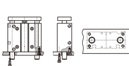
Фиксация винтами за заднюю поверхность
