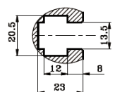
Вид на Т-образный паз
