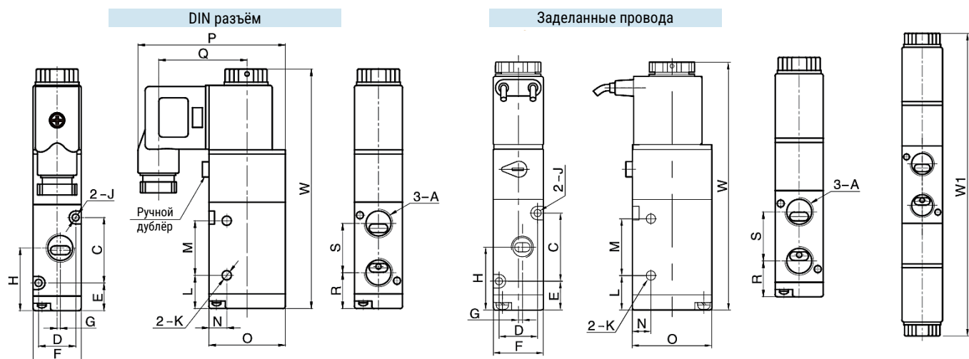
Моностабильный распределитель
