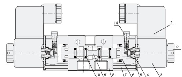
Бистабильный распределитель
